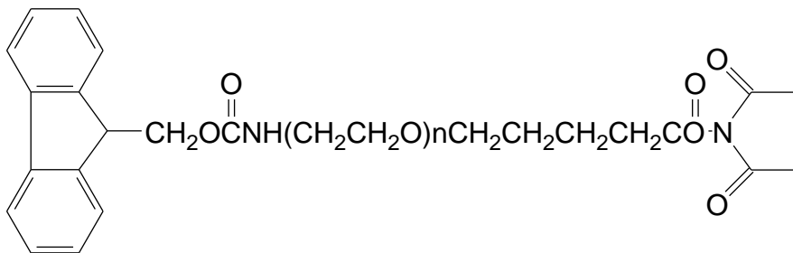
FMOC-NH-PEG-SVA
