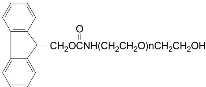
FMOC-NH-PEG-OH
