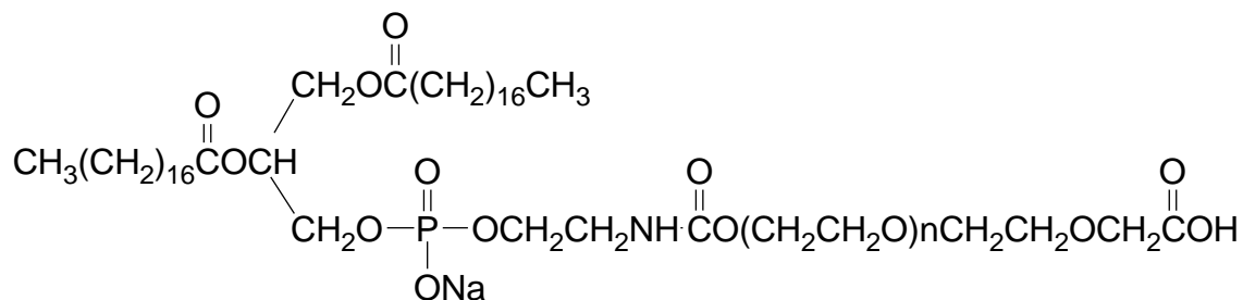
CM-PEG-DSPE
