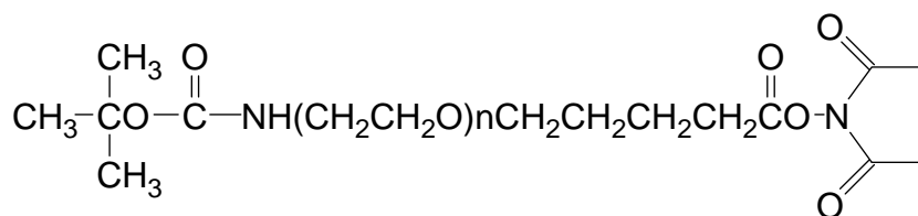
tBOC-NH-PEG-SVA
