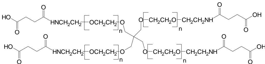
4ARM-PEG-ASA
